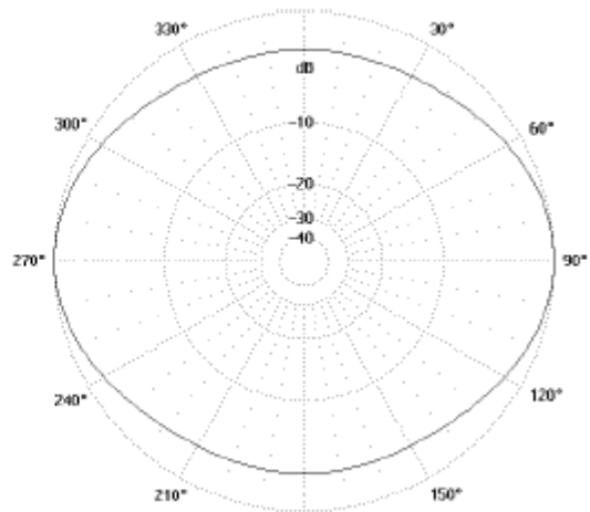
Diagramme de rayonnement plan H L'antenne est installée au sommet du mât. Fréquence d'émission 455 MHz, L = (\lambda/2) = 347 \text{ mm}^{**} Code de la caractéristique de rayonnement : 070 CA 00
