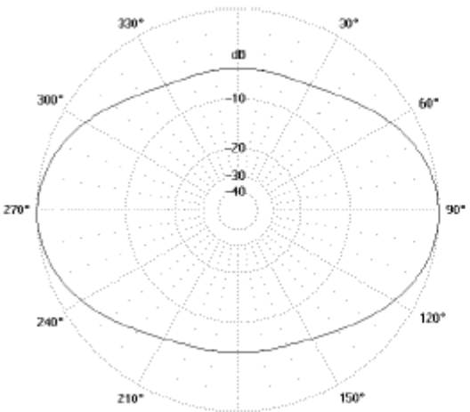
Diagramme de rayonnement plan H L'antenne est installée à mi-hauteur du mât. Fréquence d'émission 455 MHz, L = (\lambda/2) = 347 \text{ mm}^{**} Code de la caractéristique de rayonnement : 050 CA 00
