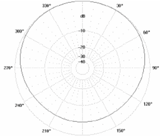
Diagramme de rayonnement plan H L'antenne est installée au sommet du mât. Fréquence d'émission 455 MHz, L = (\lambda/4) = 174 \text{ mm}^* Code de la caractéristique de rayonnement : 060 KA 00
