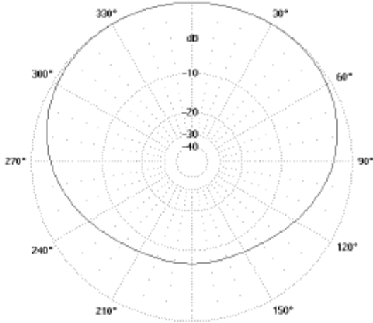
Diagramme de rayonnement plan H L'antenne est installée à mi-hauteur du mât. Fréquence d'émission 455 MHz, L = (\lambda/4) = 174 \text{ mm}^* Code de la caractéristique de rayonnement : 040 KA 00
