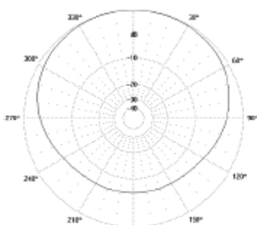
Diagramme de rayonnement plan H
